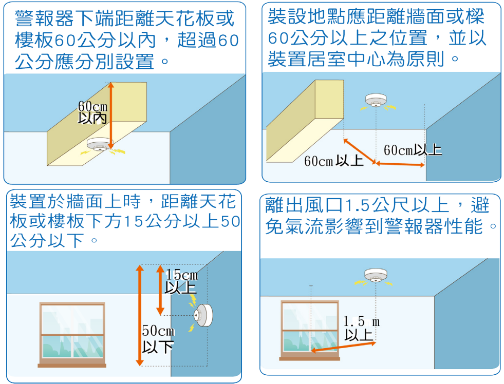
圖 4 住宅用火災警報器裝設示意圖
